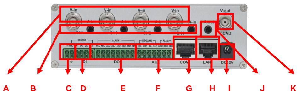
Picture 4 : FW-3450 Widok tylnego panelu
