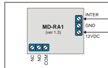
opis wyprowadzeń
