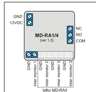
opis wyprowadzeń
