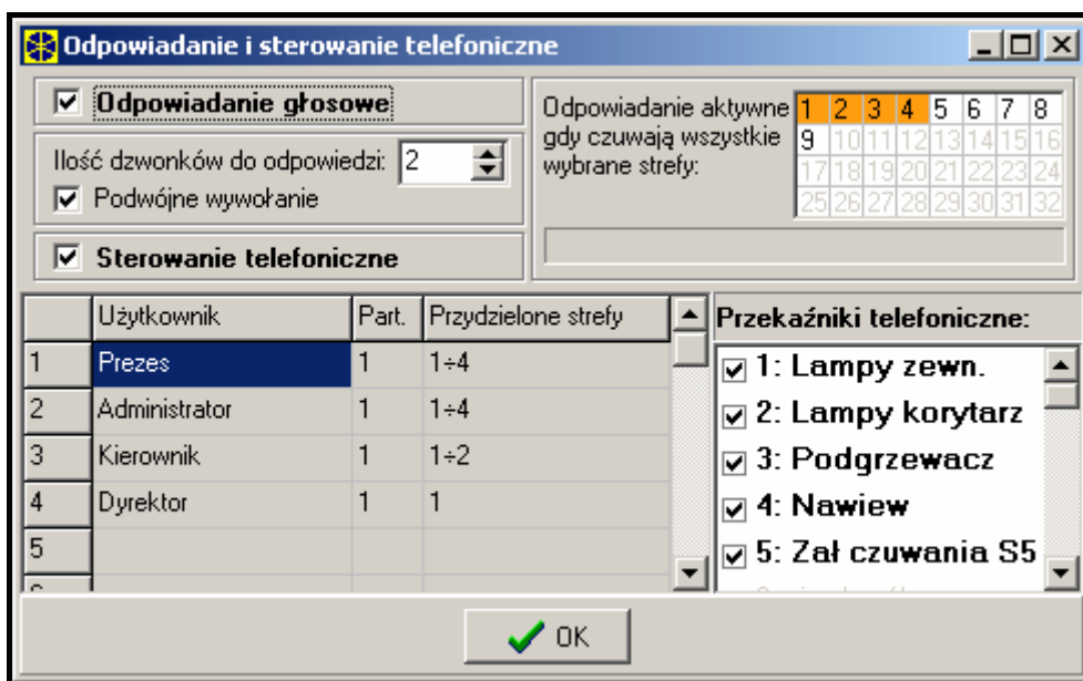
Rys. 23. Określenie, jakie przełączniki telefoniczne mogą być sterowane przez użytkowników.
